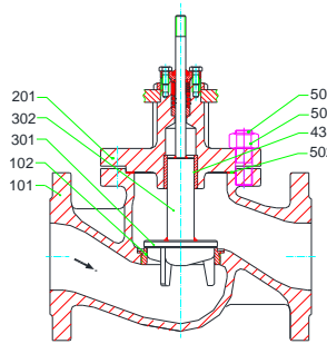
MV 5211-AR, PV 6211-AR NPS 3 - 4, CL 150 - 300
