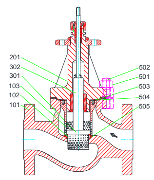
MV 5211-AR, PV 6211-AR with/ mit/ avec QCS 2-stage NPS 2½ - 3, CL 600
