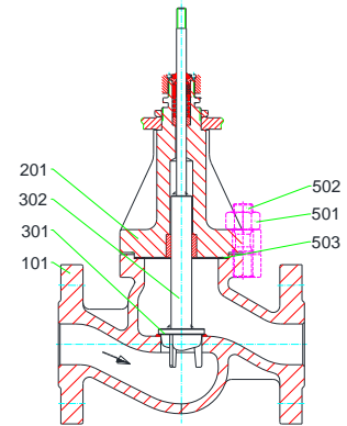
MV 5211-AR, PV 6211-AR NPS 2½ - 4, CL 600 - 900
