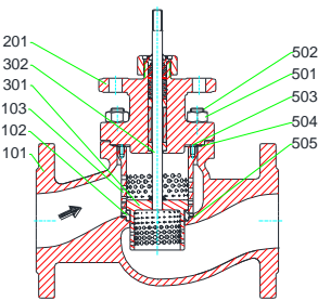
MV 5211-AR, PV 6211-AR with/ mit/ avec QCS 2-stage NPS ½ - 2½, CL 150 - 300
