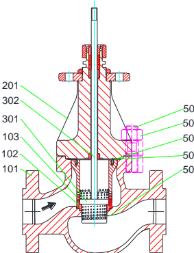
MV 5211-AR, PV 6211-AR with/ mit/ avec QCS 2-stage NPS ½ - 2, CL 600
