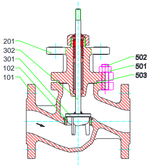
MV 5211-AR, PV 6211-AR NPS ½ - 2½, CL 150 - 300
