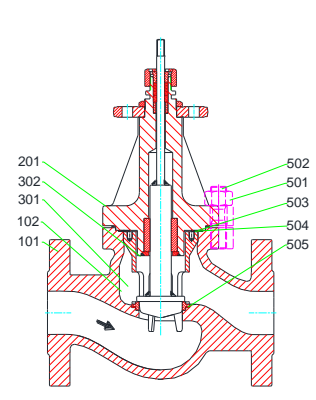
MV 5211-AR, PV 6211-AR with/ mit/ avec QCS NPS 2½ - 4, CL 600
