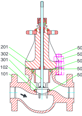
MV 5211-AR, PV 6211-AR with/ mit/ avec QCS NPS ½ - 2, CL 600
