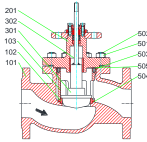
MV 5211-AR, PV 6211-AR with/ mit/ avec QCS NPS 3 - 4, CL 150 - 300
