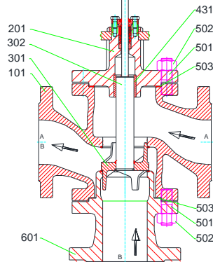
MV 5221-AR, PV 6221-AR NPS 4, CL 150 - 300
