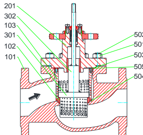
MV 5211-AR, PV 6211-AR with/ mit/ avec QCS 2-stage NPS 3 - 4, CL 150 - 300
