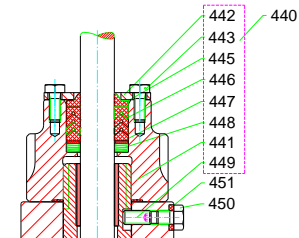
NPS ½ - 4, CL 150
