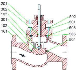
MV 5211-AR, PV 6211-AR with/ mit/ avec QCS NPS ½ - 2½, CL 150 - 300
