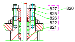
DN 80-150, PN 16-40
