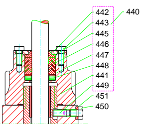
DN 20-150, PN 16-25
