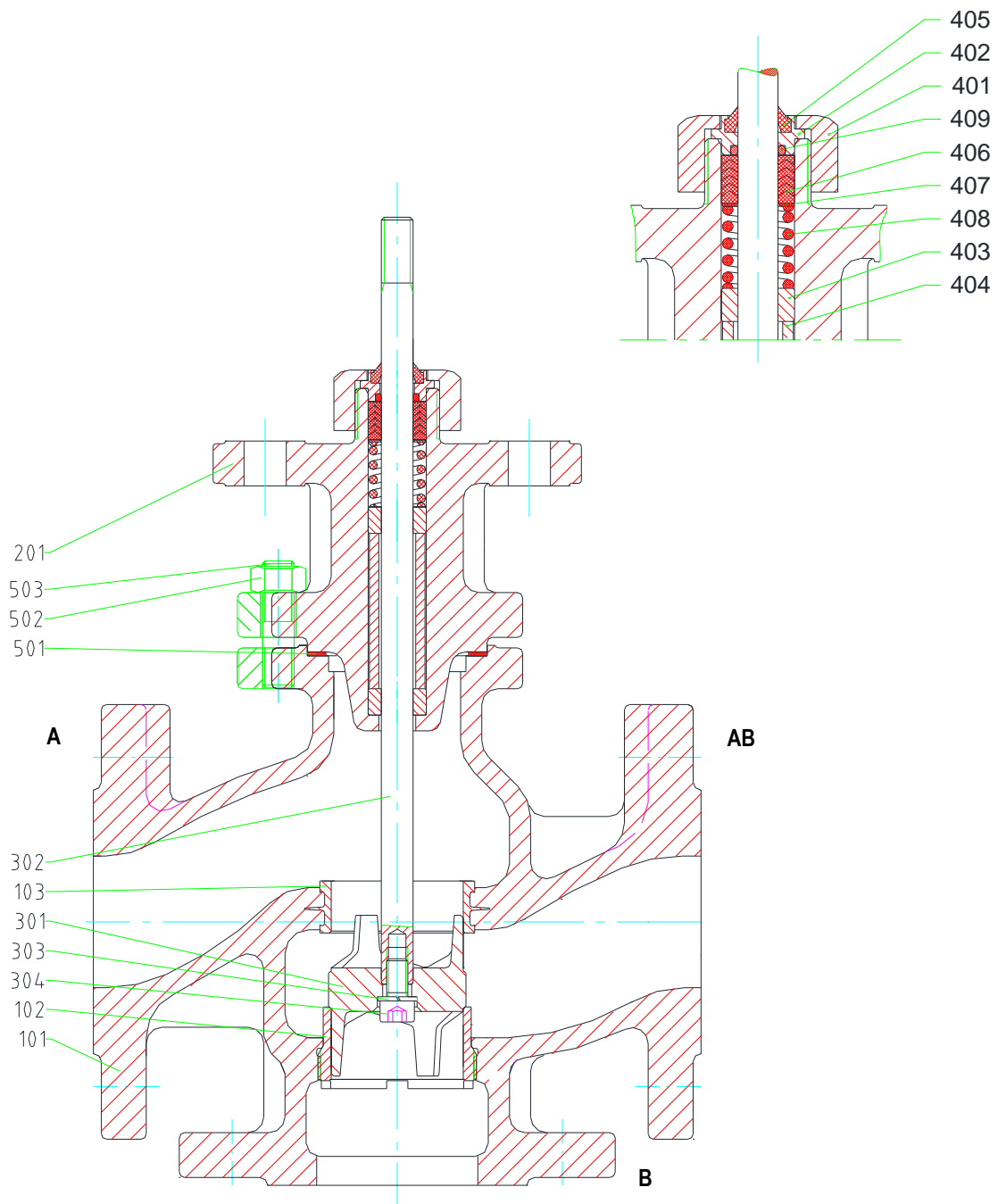
MV 5271 / PV 6271, PN 16,25
