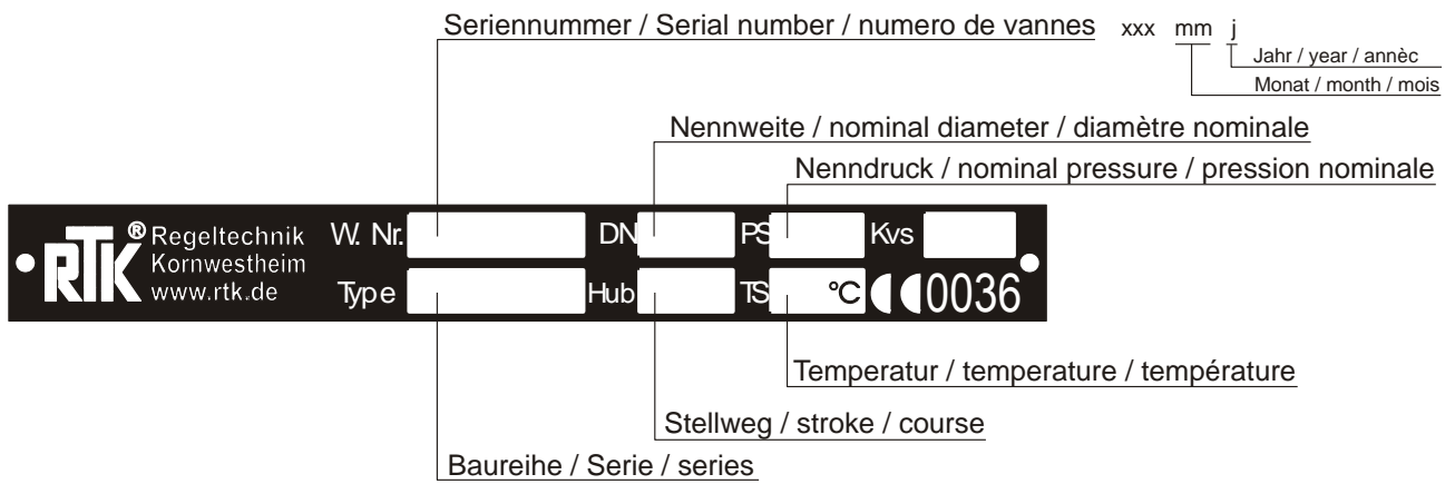
Bild 1/ Figure 1 : Typenschild auf Ventil / nameplate on valves /
