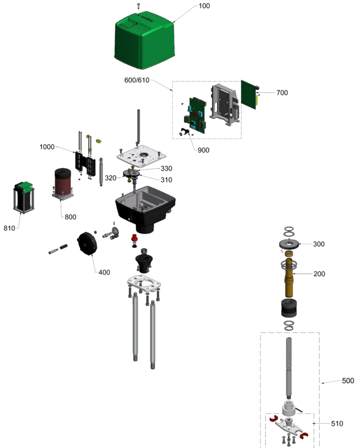
REact 60_100 mit Säulen / with pillars / avec colonnes
